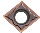
CCMT 060204/08 CCMT 09T304/08 CCMT 120404/08
