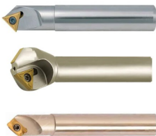
CHAMFER TOOL 30°, 45°, 60°
